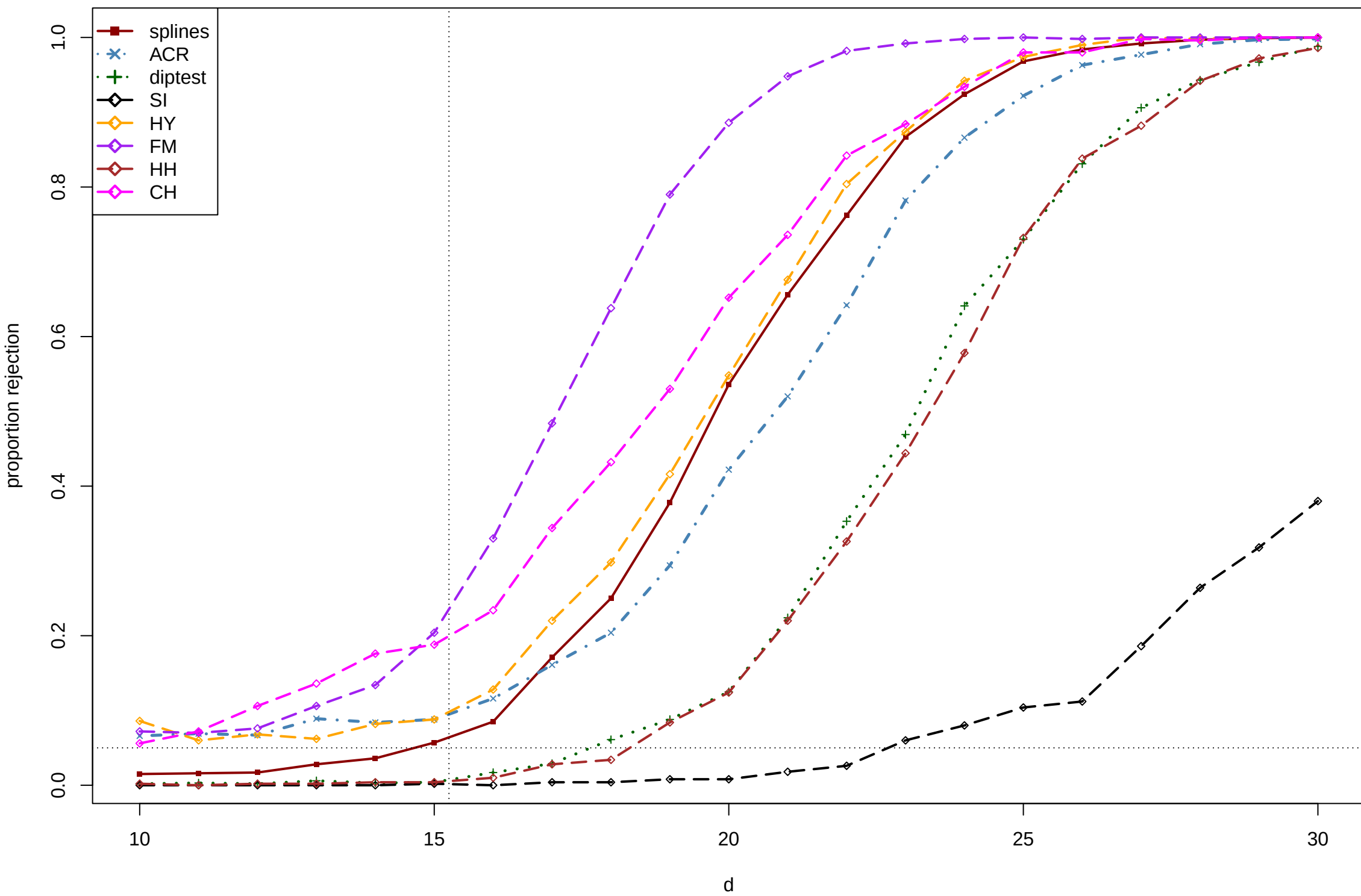
0.5chisq(5)+0.5chisq(d), n=200
